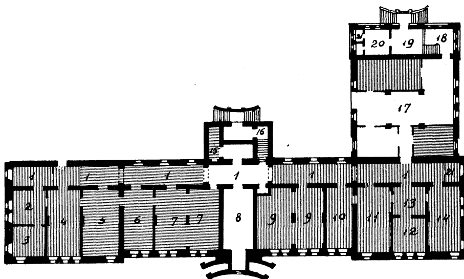
FIG. III. - Pianta sotterranea.
