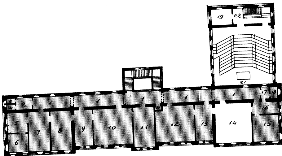
FIG. V. - Primo piano.
