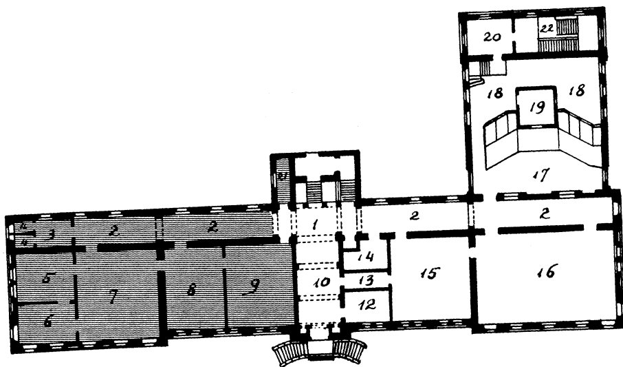
FIG. IV. - Pianoterra rialzato.
